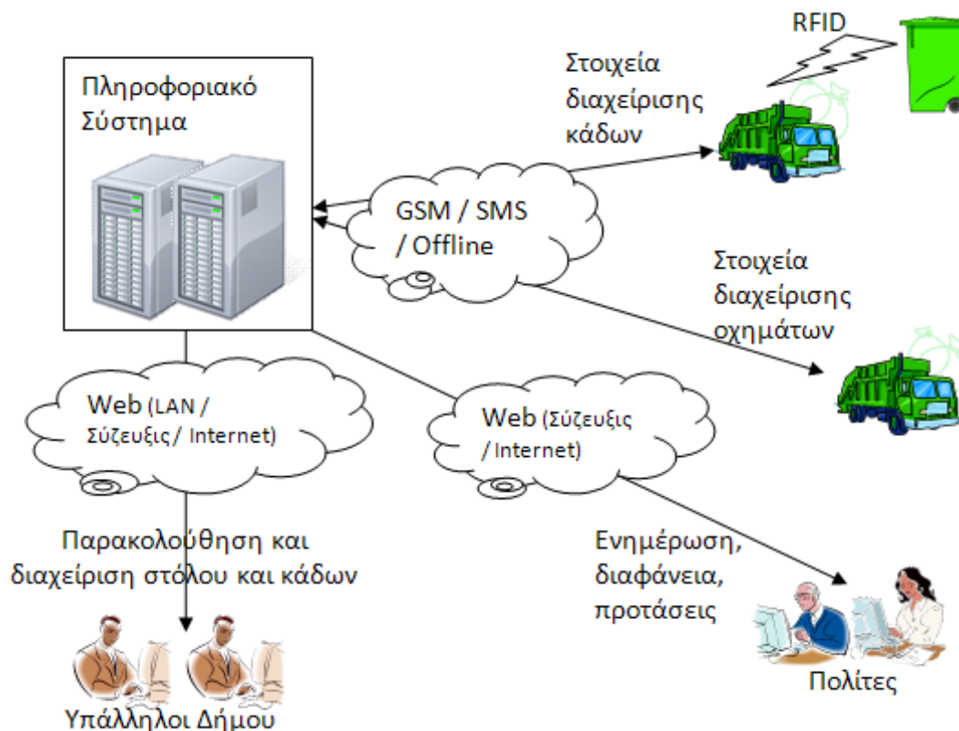
Εικόνα 1: Λειτουργική Αρχιτεκτονική Συστήματος
